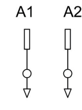
E 型 (负载无极性)
